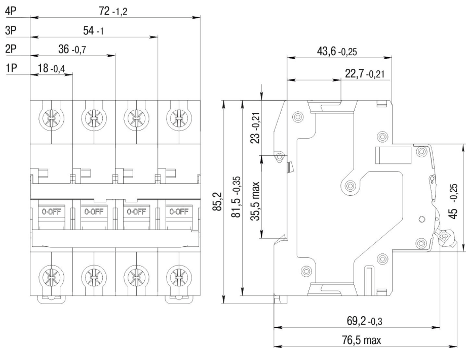
Рисунок 1. Габаритные и установочные размеры
