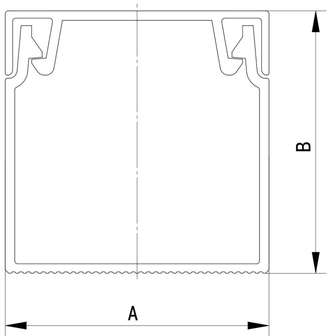
Рисунок 1. Габаритные размеры кабель-канала
