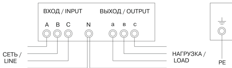
Рисунок 1 – Схема подключения СНИЗ-3 кВА
