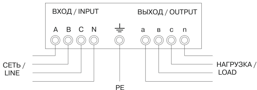
Рисунок 3 – Схема подключения СНИЗ от 15 до 60 кВА
