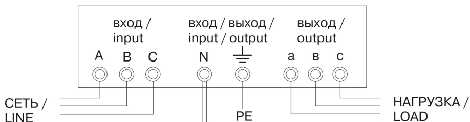
Рисунок 2 – Схема подключения СНИЗ от 6 до 7,5 кВА
