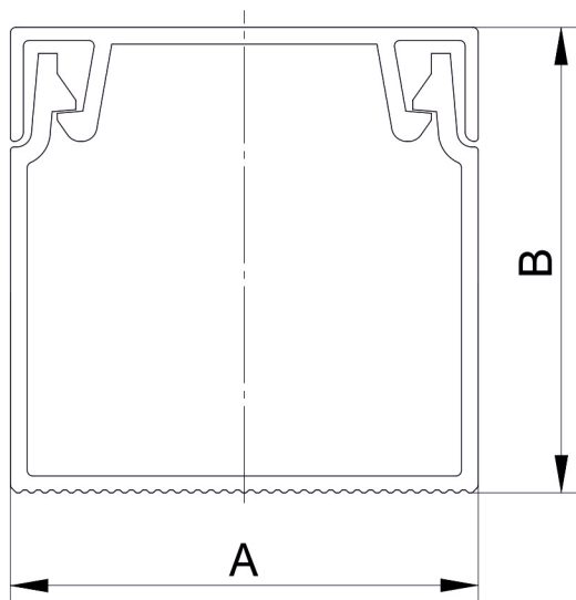
Габаритные размеры и площадь внутреннего поперечного сечения
