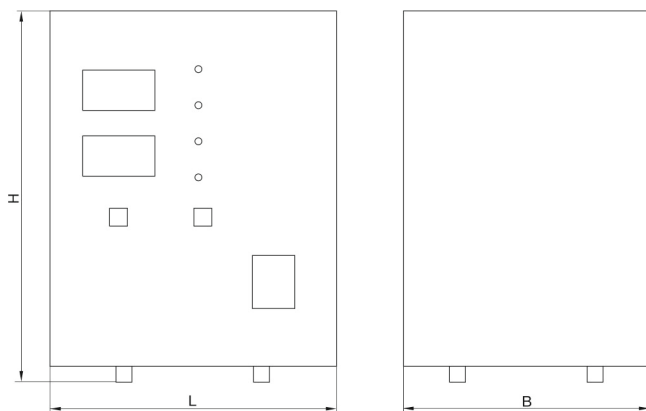
Рисунок 1 – Габаритные размеры:
